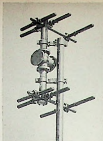
Bild 4. Eine der drei Ballemfangsantennen (im Bild: die verstellbare, witterungsfeste Ausführung für Band III)
