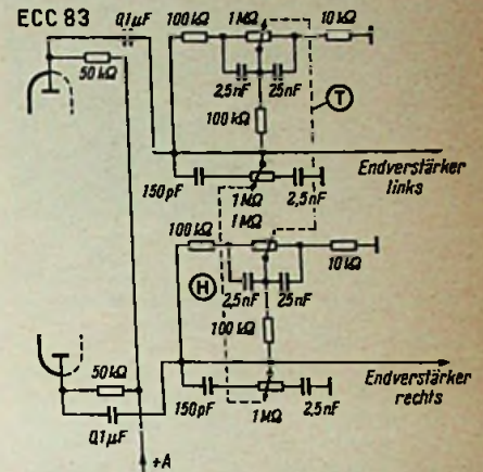
Bild 8. Doppelseitig wirkendes Stereo-Klangregel-Netzwerk
