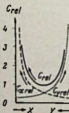
Rechts: Bild 2. Abhängigkeit der Kapazität von den Plattenabständen bzw. der Lage des Rotors
