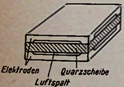
Links: Bild 4. Alterer Quarzaufbau: Quarzscheibe (Dickens-Scherschwingen) zwischen zwei Elektroden mit Luftspalt
