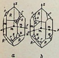
Bild 1. Die ideale Quarzgeometrie, a) Rechtsquarz, b) Linksquarz
