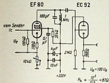
Bild 7. Hilfsschaltung zum Erzeugen genügend großer Eichspannungen
