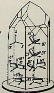
Bild 2. Wie die verschiedenen Quarzschnitte im Quarzkristall liegen
