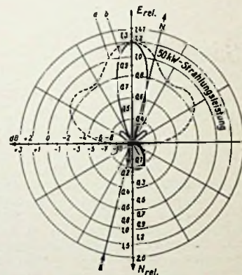
Bild 7. Strahlungsdiagramm der UKW-Rundfunkantenne in Band II; a) horizontal, b) vertikal
