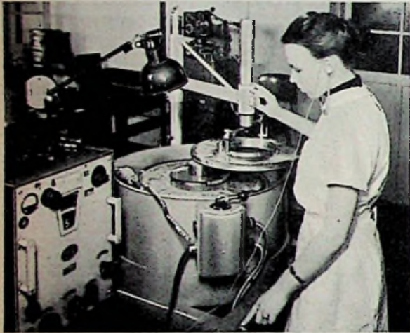
Bild 3. Läppmaschine [geöffnet] mit angeschlossenen Empfänger für die Frequenzüberwachung in der Quarzfertigung der C. Lorenz AG
