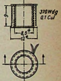
Bild 2. Bau- und Wickelskizze der Entzerrer-Drossel
