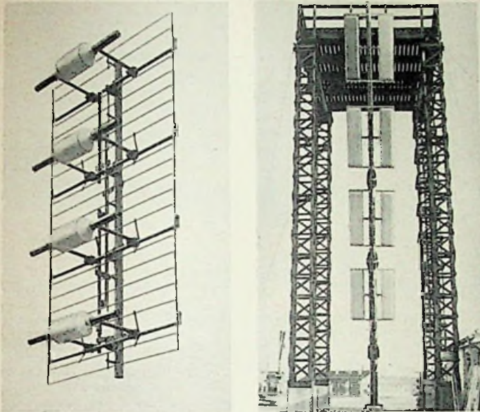
Bild 1. Breitband-Dipolfeld für Band III. Vier solche Felder bilden die Nord- und eines bildet die Südantenne des Fernsehenders auf dem Säntis
