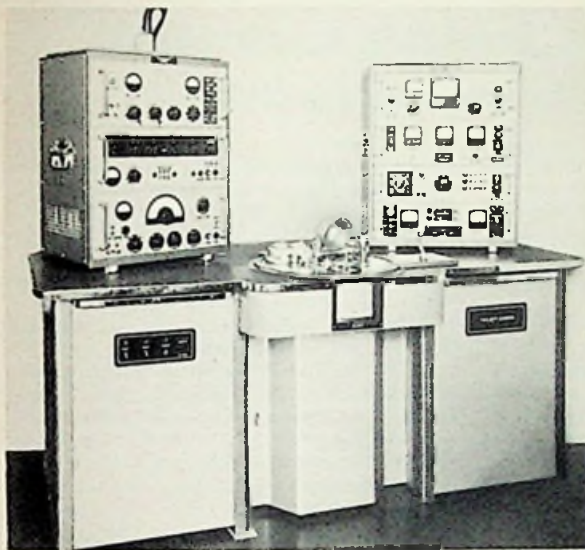
Bild 8. Gesamtansicht der in Bild 7 skizzierten Aufdampfanlage. In der Mitte Drehtisch mit drei Rezipienten, links Präzisionsfrequenzmesser 1 kHz...300 MHz, Genauigkeit 1 \cdot 10^{-7} , rechts Automatik, im Tisch Vakuumpumpen und Stromversorgung
