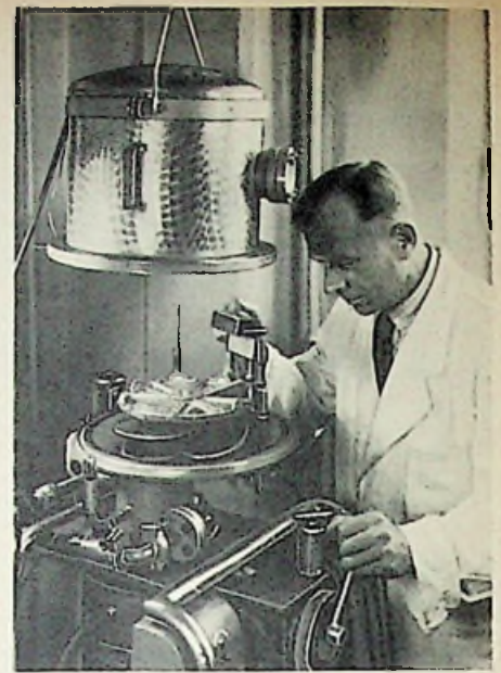
Bild 6. Aus der Schwingquarzfertigung bei Siemens: Aufbringen der Schichtelektroden im Vakuum-Pumpstand mit Katodenzerstäubung
