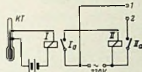
Bild 2. Schaltanordnung zur Temperaturregelung. KT = Kontaktthermometer, das möglichst in unmittelbarer Nähe der Transistoren zu montieren ist. I = Feinrelais, in Arbeitsstellung gezeichnet, II = Schaltschütz. 1, 2 = Anschlüsse für den Wärmestrahler
