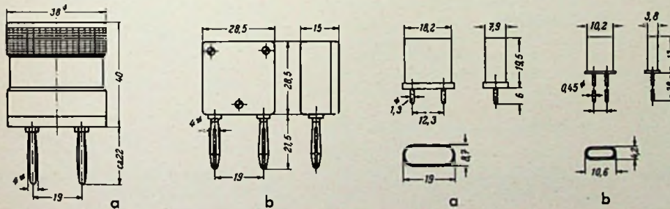
Bild 10. Maßskizzen von Preßstoffhaltern (Dr. Steeg & Reuter). a) ältere runde Form, b) neuere flache Form
