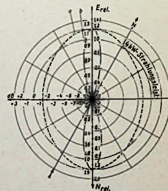
Bild 8. Strahlungsdiagramm der Autorufantenne
