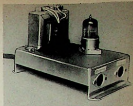
Bild 4. So sieht das selbstgebaute Hilfsgerät für Stereo-Kopfhörer-Wiedergabe aus
