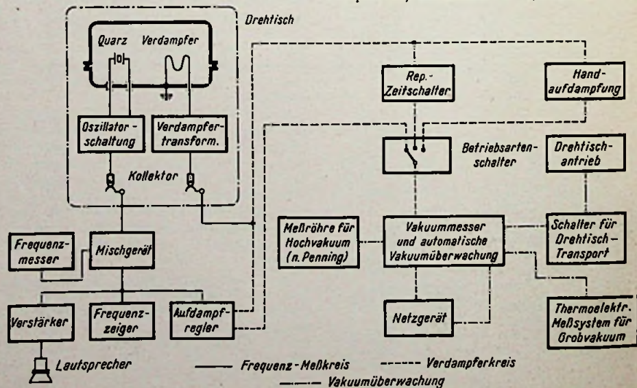
Bild 7. Blockschaltbild der von Telefunken entwickelten Quarz-Aufdampfanlage
