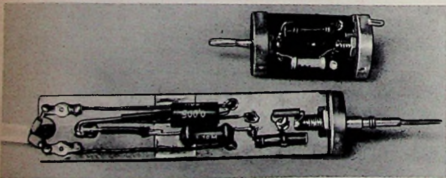
Bild 5. Innen-Anordnung des Tastkopfes und des Aufsteck-Spannungsteilers. Die Verbindungen werden durch eingelötete Messing-Hohlknoten gehalten
