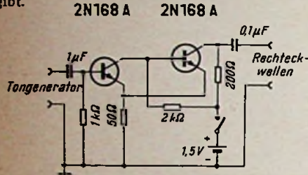
Schaltung eines Schmitt-Triggers, der vom Tongenerator gesteuert wird
