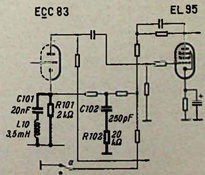
Bild 1. Die erforderlichen Änderungen der Originalschaltung sind stark eingekreist
